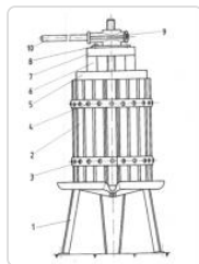
Sulčiaspaudės bendras vaizdas ir dalių schema
