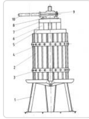
Sulas spiedes vispārējais skats un detaļu shēma
