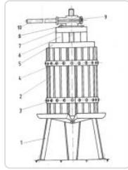
Mahlapressi üldvaade ja osade joonis
